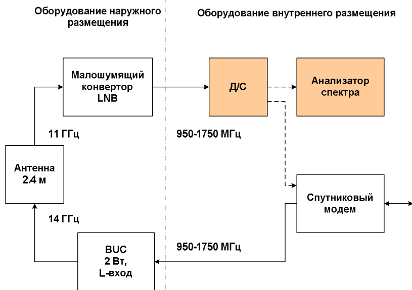
Рисунок 10 - Типовая структурная схема ЗС с анализатором спектра для первоначального наведения антенны на КА (вариант 1)
