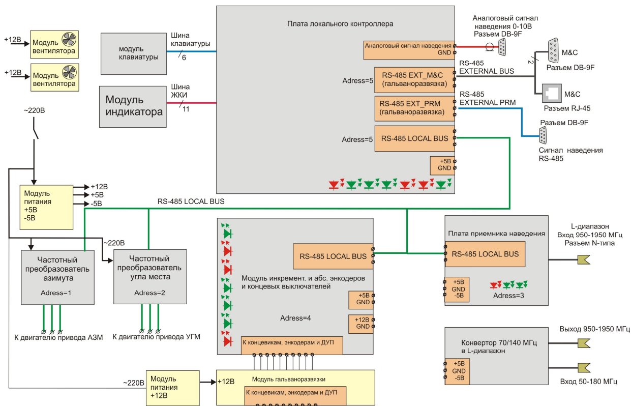
Рисунок 5 - Структурная схема БУА модель 3700
