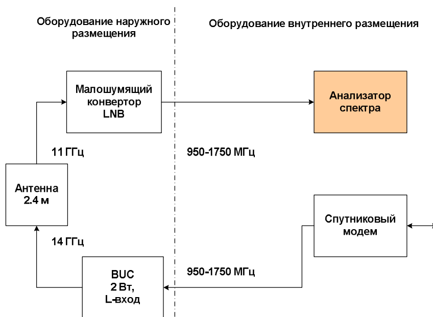
Рисунок 11 – Типовая структурная схема РС с анализатором спектра для первоначального наведения антенны на КА (вариант 2)
