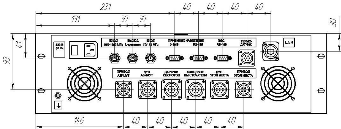
Рисунок 4 - БУА, задняя панель. Габаритные и установочные размеры
